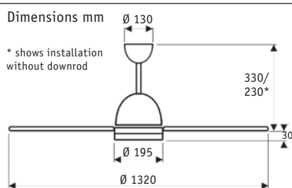
LIBELLE 132
